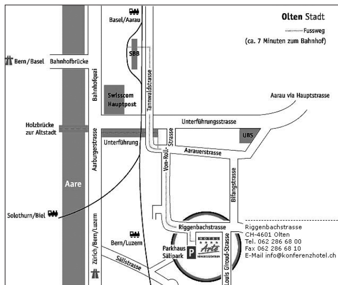
Anfahrtskizze
